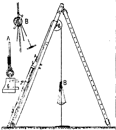
Č. 530. Beranidlo tahací.
